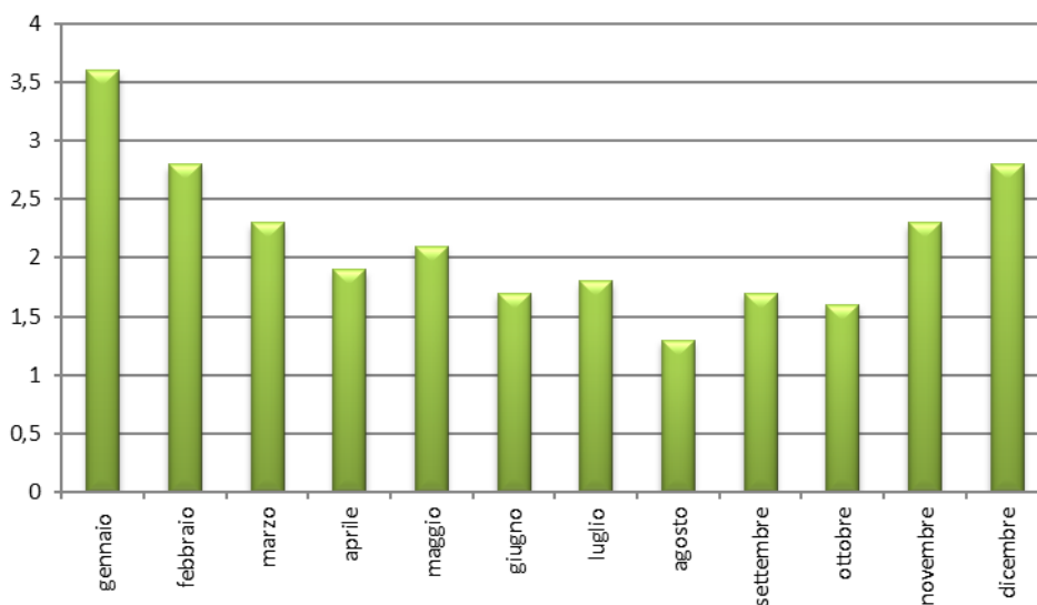
Figura 23 – Velocità del vento medie mensili registrate (m/s) – 2024
