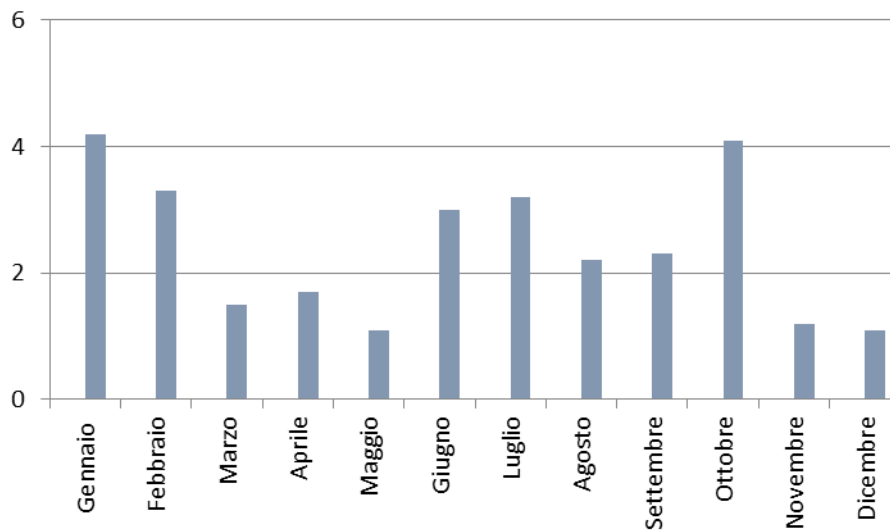
Figura 14 - Andamento delle concentrazioni medie mensili di Nichel in ng/m 3 nel periodo considerato – 2024
