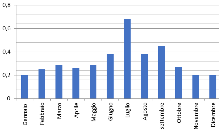
Figura 10 - Andamento delle concentrazioni medie mensili di ARSENICO in ng/m 3 nel periodo considerato – 2024
