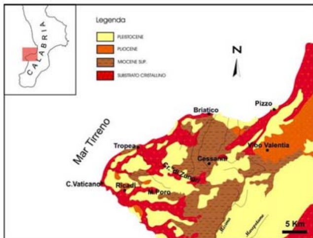
Fig. 1 - Inquadramento geografico e geologico del Monte Poro (VV). - Geographical and geological framework of Monte Poro (VV).
